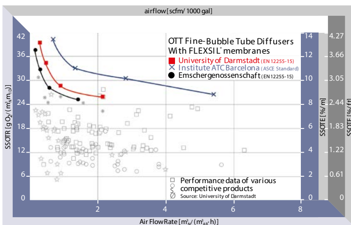
Los difusores para tuberías de membrana de OTT garantizan la aireación de las burbujas finas.
